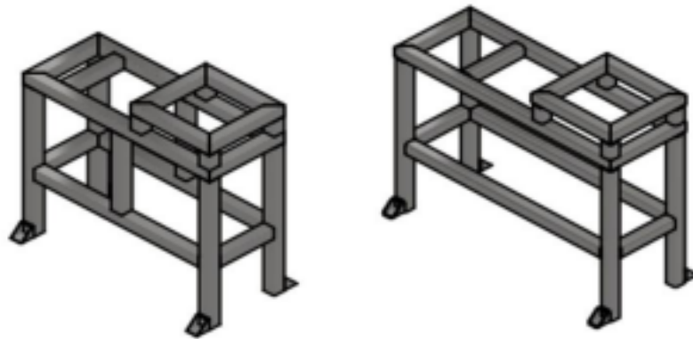
Gambar 5 Bagian Rangka Referensi Desain (kiri) dan Modifikasi Desain (kanan)
