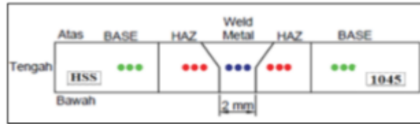
Gambar 15 Posisi daerah pengujian kekerasan.
