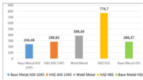
Gambar 17 Nilai kekerasan rata-rata pada amper \pm 273A .
