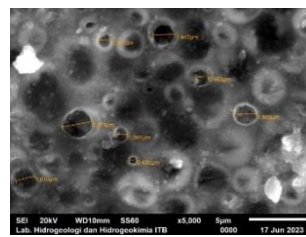
Gambar 5. Morfologi Tampak Samping Membran Polisulfon-Kitosan Sesudah Filtrasi
