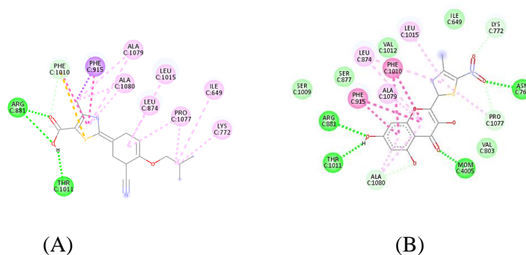
Gambar 4. Interaksi senyawa Febuxostat (A) dan Ligan Uji 5 (B) dengan reseptor xantin Oksidase.
