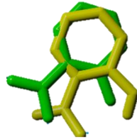
Gambar 1. Posisi tumpang tindih ligan native dari struktur reseptor kristal sinar x (hijau) dengan ligan native hasil redocking (kuning).
