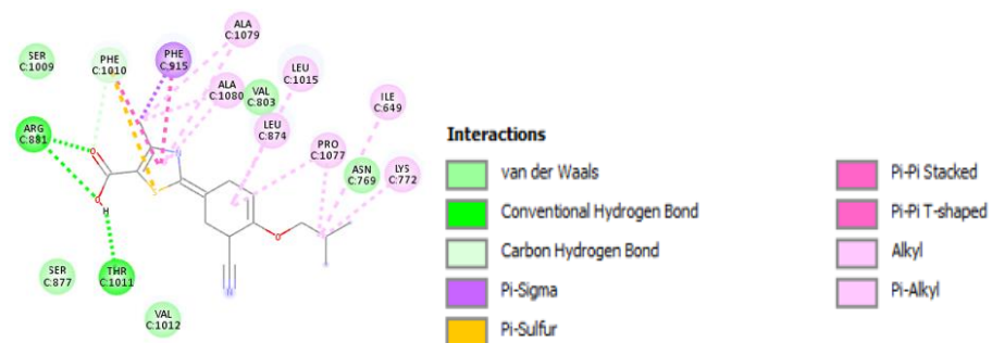
Gambar 2 Interaksi febuxostat dengan reseptor enzim xantin oksidase
